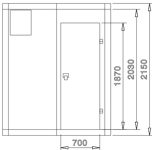
Zepředu
